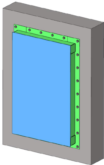
防護板 (既設窓部へ設置)
