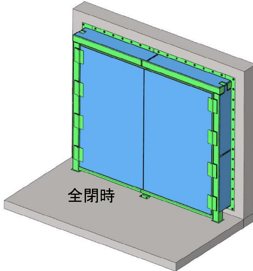
防護扉(既設扉部へ設置)
