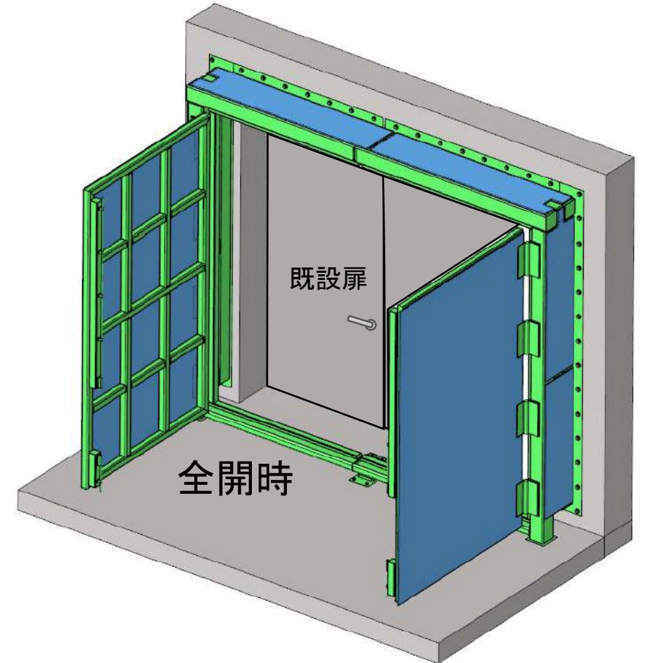
防護扉(既設扉部へ設置)
